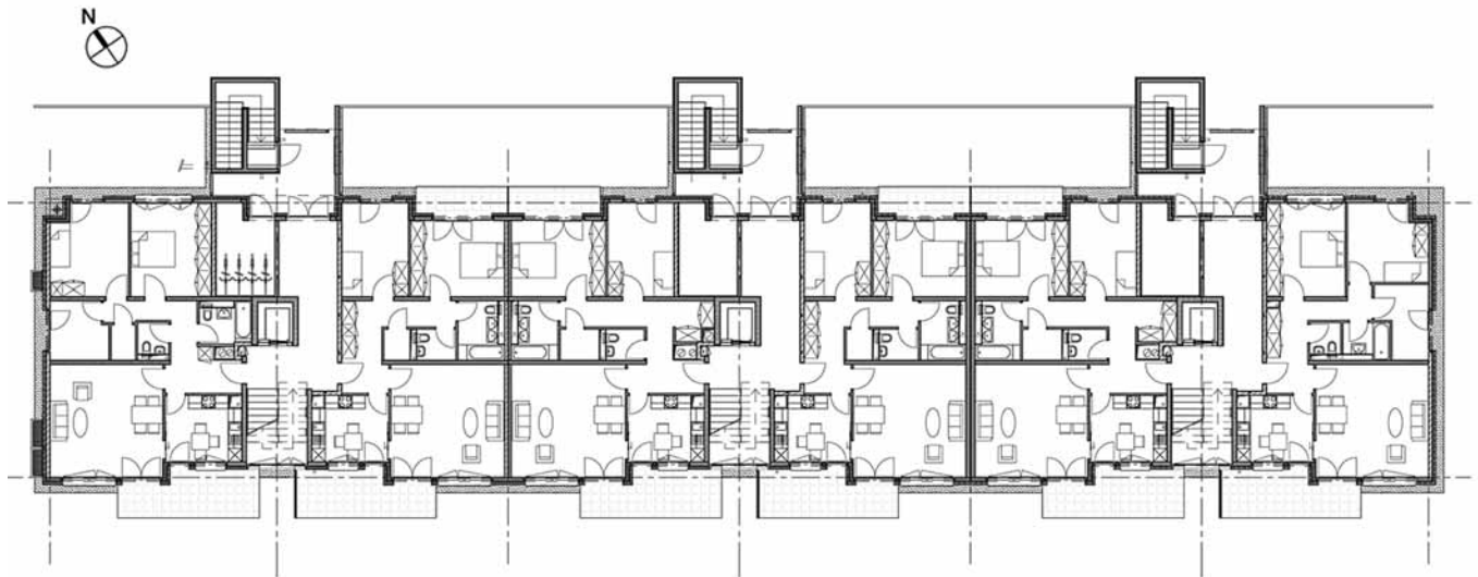
Bâtiment B, plan du rez-de-chaussée
