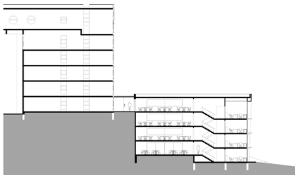
Coupe transversale
